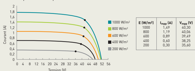
La puissance dépend de l'ensoleillement Modèle de module SCG60-HV-F
