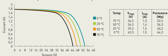
Courbes de puissance à différentes températures Modèle de module SCG60-HV-F
