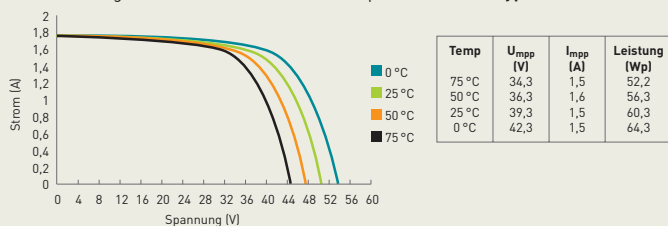
Leistungskurven bei verschiedenen Temperaturen Modultyp SCG60-HV-F
