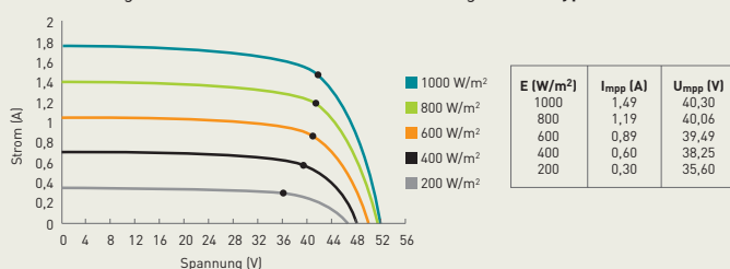
Leistungskurven bei verschiedenen Einstrahlungen Modultyp SCG60-HV-F
